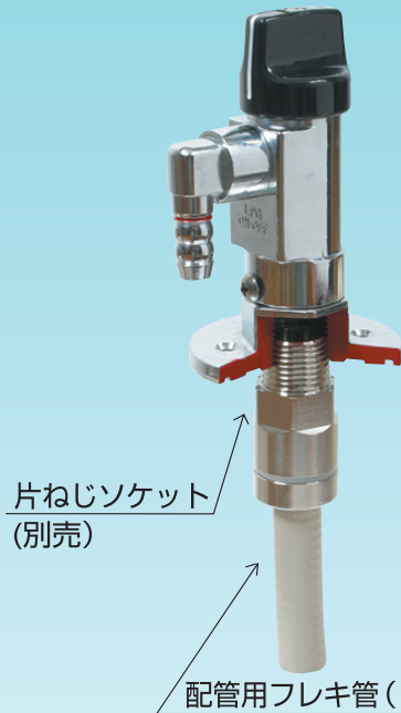
■ GPL-6FOFFP・Rc \frac{1}{2}
